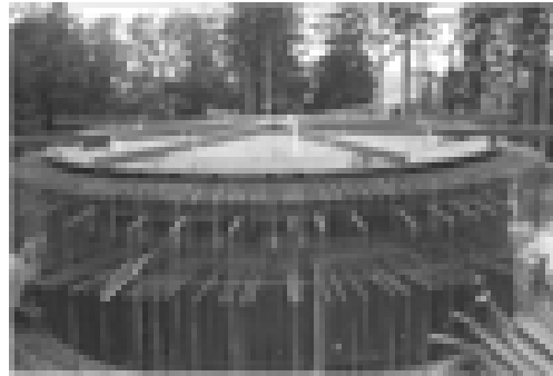
Fundament des neuen Windrads Foto: Leimer
